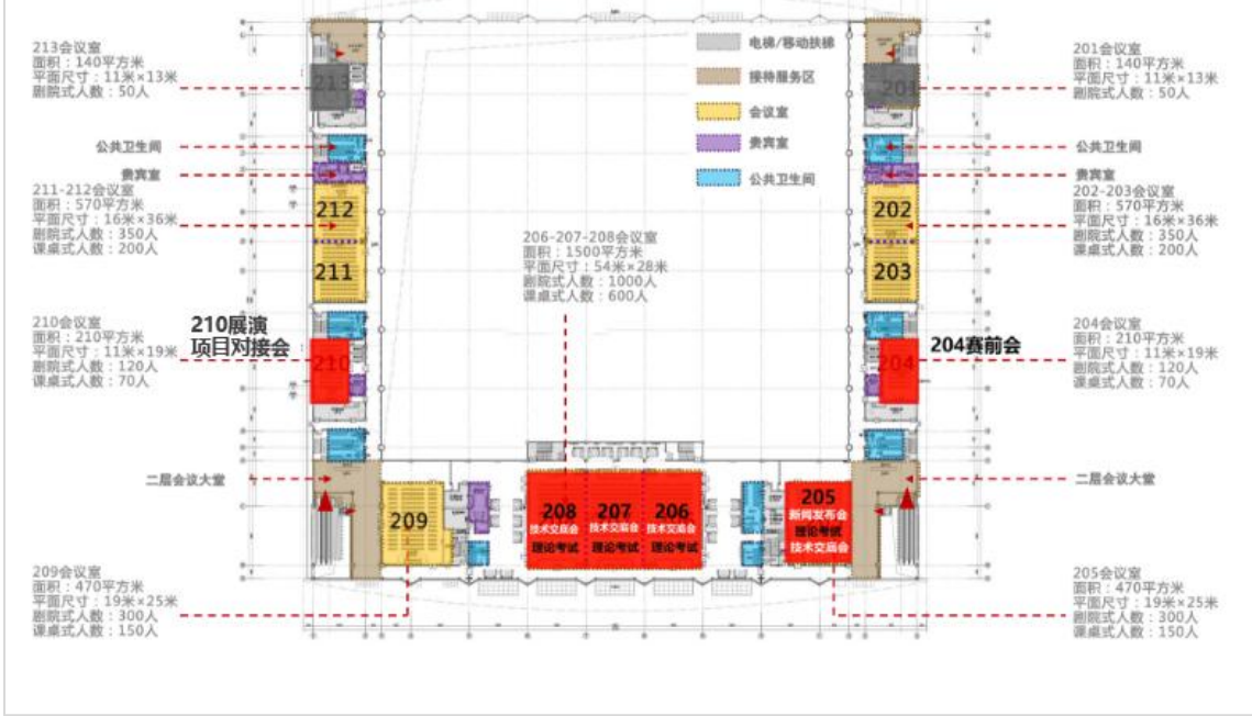
合肥滨湖国际会展中心西区会议厅平面图
